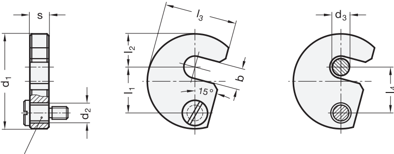
Flat shoulder screw DIN 923
