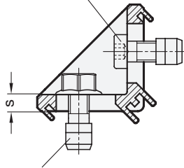
Assembly set for slot width 10 2x T-Slot bolt GN 505.4 2x Flange nut DIN 6923
