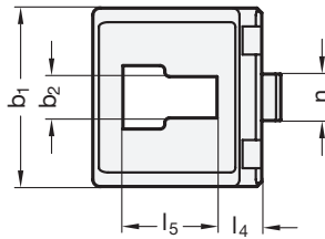
Assembly set for slot width 10 2x T-Slot bolt GN 505.4 2x Flange nut DIN 6923
